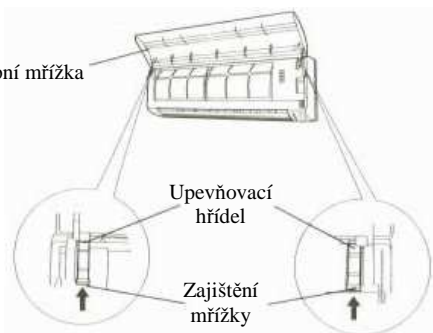
Zajištění mřížky
